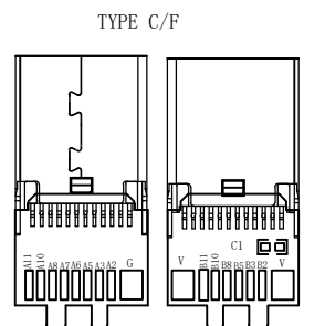
TYPE C3.1 母头焊接面
