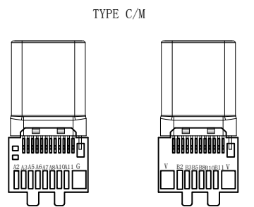
TYPE C3.1 公头焊接面
